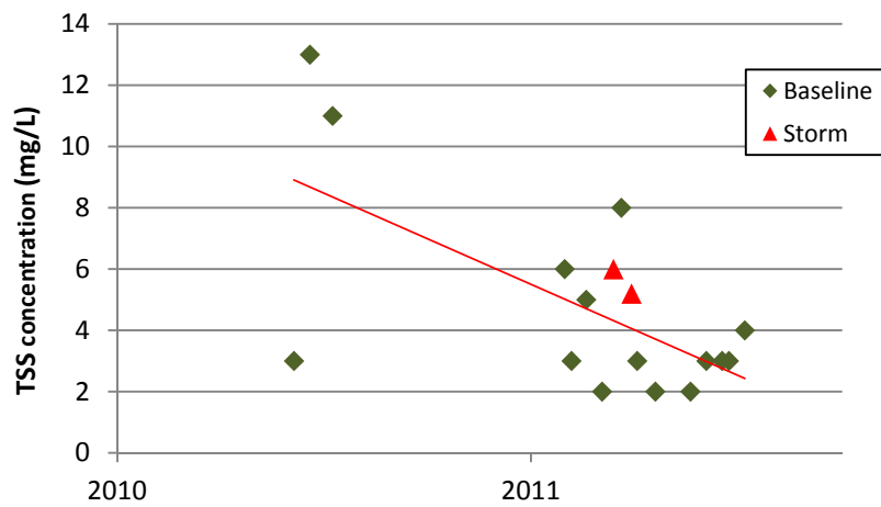
TSS @ S. Ore Creek - Third St.
