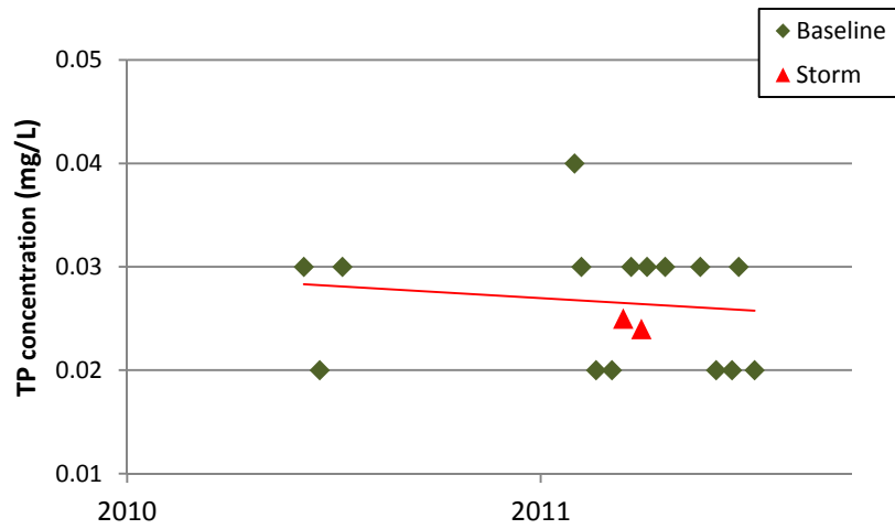
TP @ S. Ore Creek - Third St.
